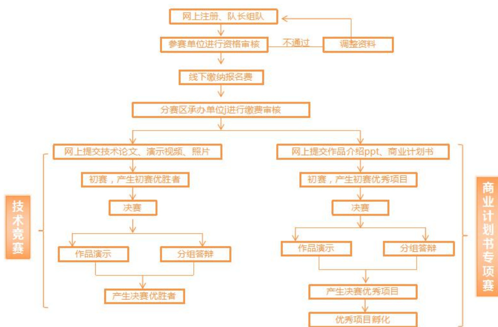
参赛流程图
